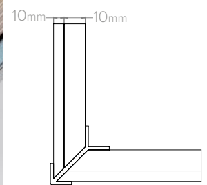
Schéma
